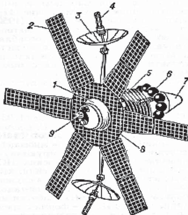
• ИСЗ «Молния-1»: 1 – герметичный корпус; 2 – панель солнечной батареи; 3 – остронаправленная антенна; 4 – датчик ориентации антенны на Землю; 5 – радиатор-холодильник; 6 – шары-баллоны с рабочим телом для проведения малых коррекций; 7 – корректирующая двигательная установка; 8 – панель нагревателя; 9 – датчик солнечной ориентации.
