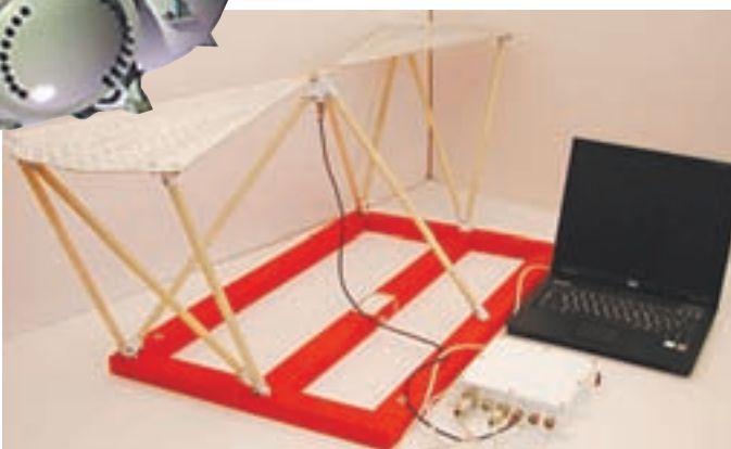
● Длинноволновый планетный радар, предназначенный для выявления глубинной структуры пород спутника планеты Марс Фобоса.
